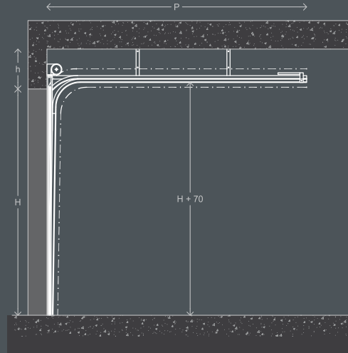
Tip. ABG - portone standard doppia guida
